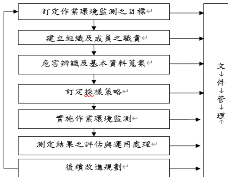
圖 1 作業環境監測計畫架構圖
